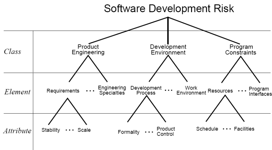
Figura 2 Clasificación de los elementos de la taxonomía del software
